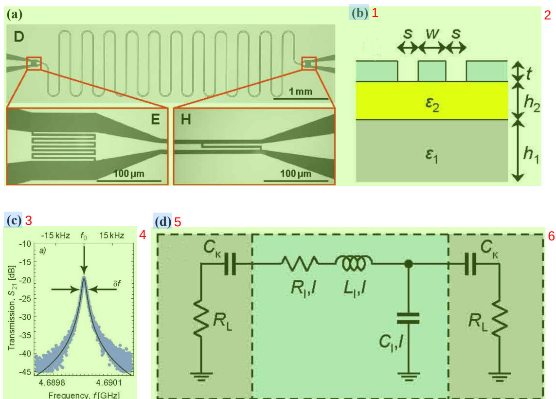
图 2.1 CPW 谐振腔结构、信号响应及等效电路图
