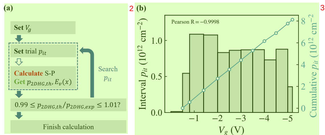
图 4.5 界面电荷填充模拟
