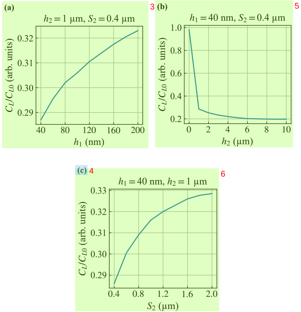
图 6.4 镂空腔参数扫描电容仿真结果 7
