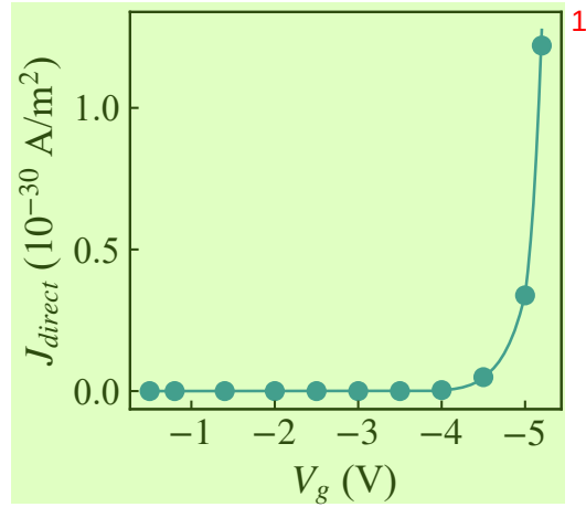
图 5.2 直接隧穿电流密度随栅压的变化
