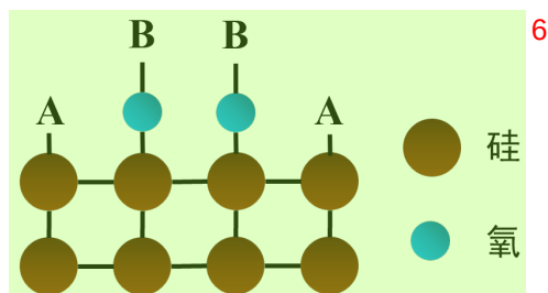
图 1.4 悬挂键示意图（以氧化硅为例）
