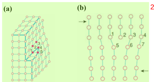
图 1.3 位错滑移示意图
