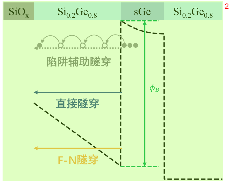
图 5.1 应变锗异质结中隧穿机制示意图
