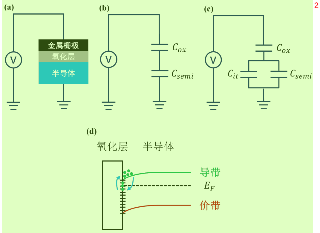
图 2.3 电容-电压法提取界面态示意图 3
