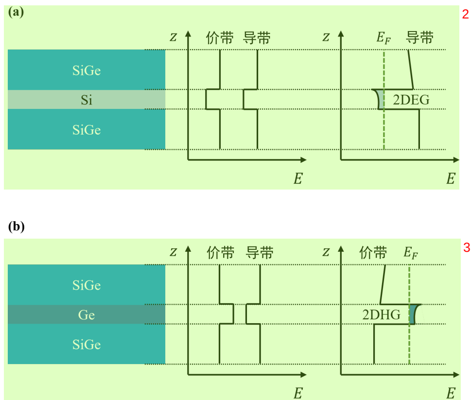
图 1.1 硅锗异质结中的载流子
