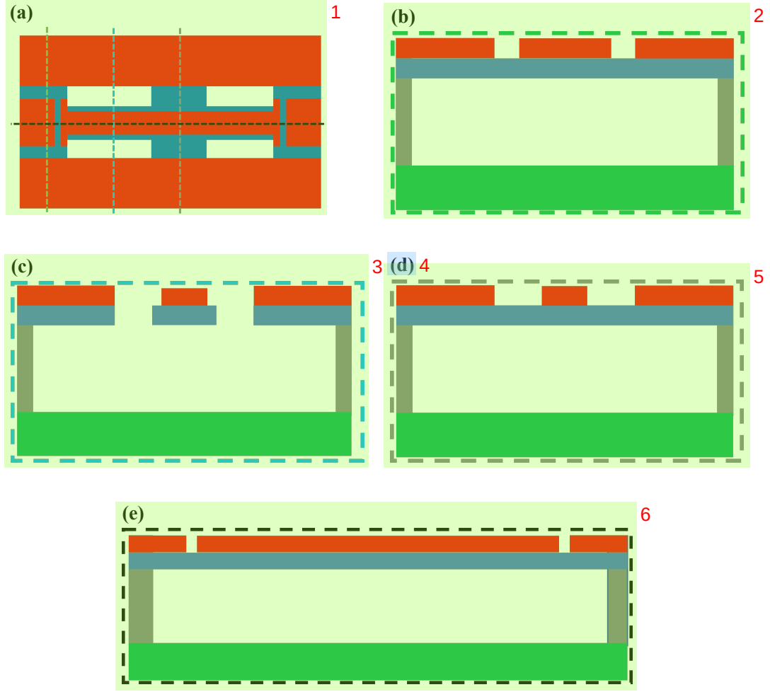
图 6.2 完整的镂空腔结构示意图 7
