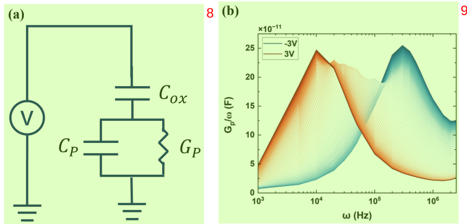
图 2.4 电导-电压法提取界面态示意图 10
