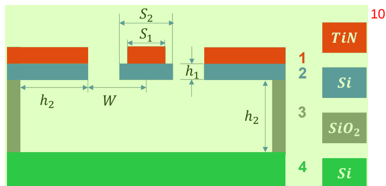
图 6.3 谐振腔仿真参数示意 11
