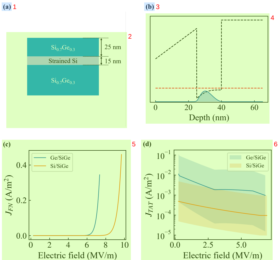
图 5.6 应变硅中隧穿电流计算结果 7
