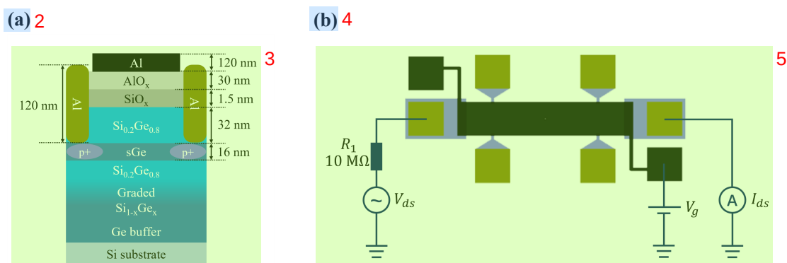
图 3.6 Hall-bar 场效应管器件与测量电路
