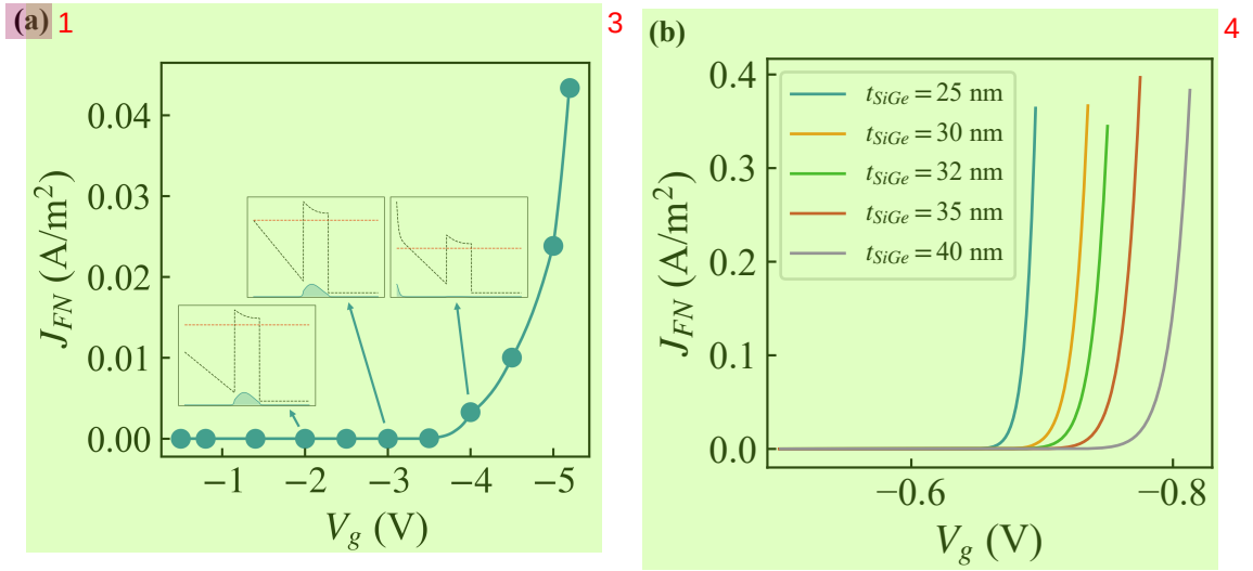
图 5.3 F-N 电流密度随栅压的变化 5
