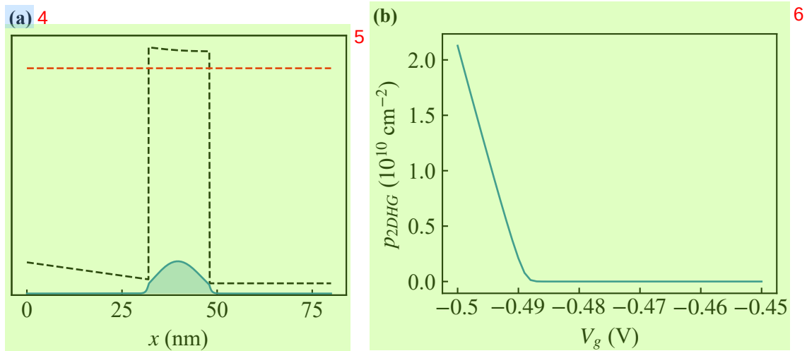
图 4.3 薛定谔-泊松求解结果示例 7
