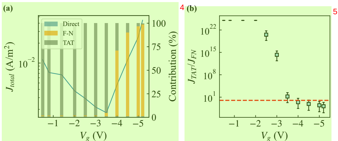
图 5.5 总体电流密度随栅压的变化 6
