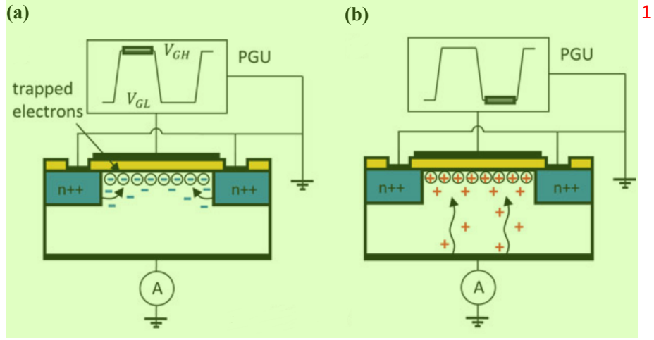
图 2.5 电荷泵浦法测量示意图
