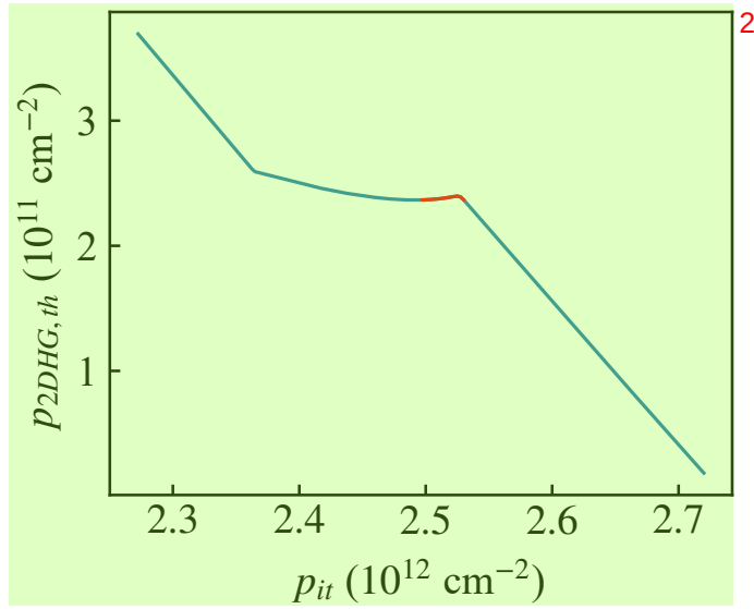
图 4.4 逆向 S-P 计算敏感性分析 3
