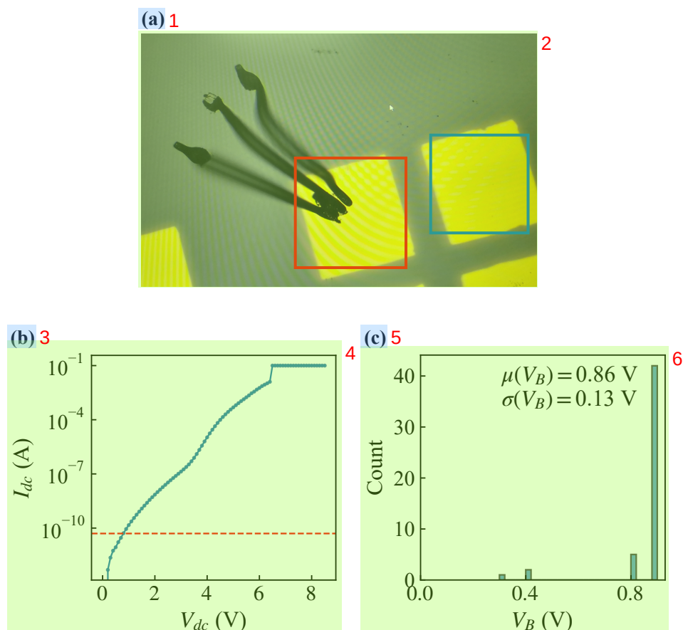
图 3.1 氧化铝击穿电压提取-300 摄氏度生长
