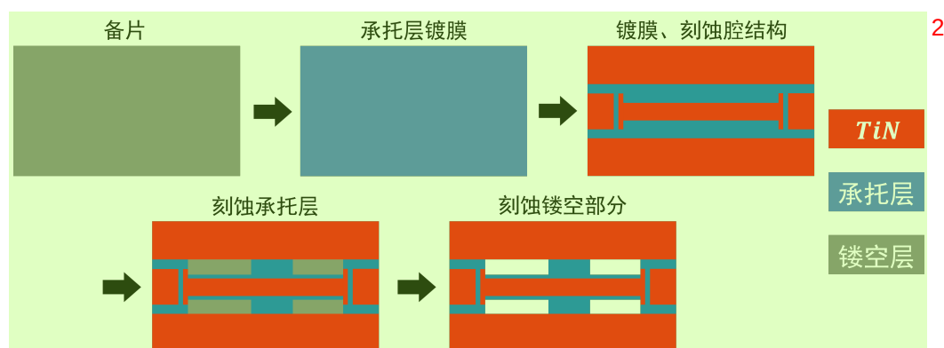
图 6.1 镂空腔制备工艺示意图
